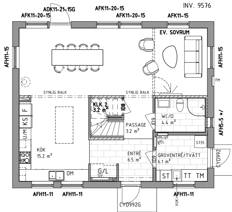
ENTRÉVÅNING
