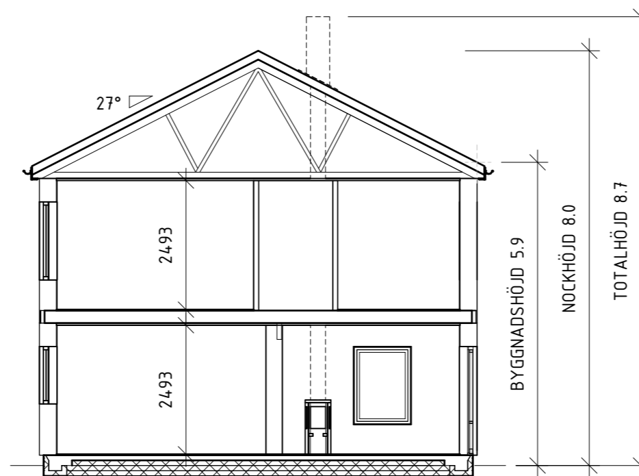
SKÅNETAKFOT SEKTION
