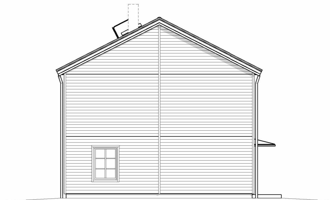
FASAD VÄNSTERSIDA
