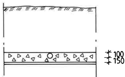
SLITSAT MARKAVLOPPSRÖR Ø110 (EJ SKALENLIG)
