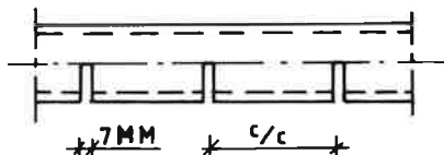
SLITSAT MARKAVLOPPSRÖR Ø110 (EJ SKALENLIG)
