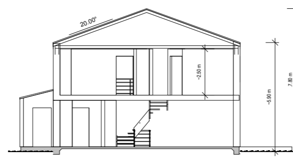
Principsektion.
