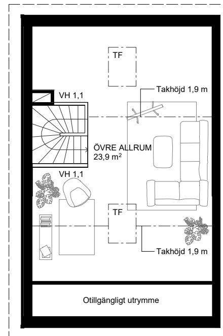
Vindsplan
