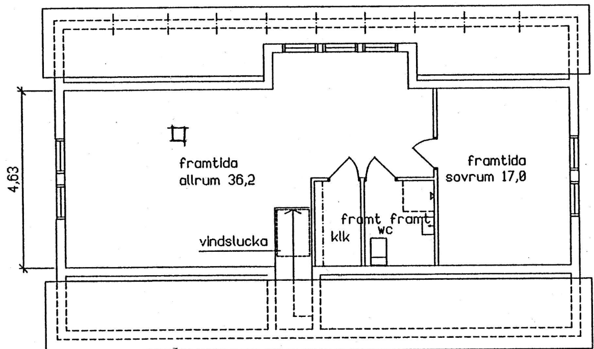
VINDSPLAN EJ INREDD (vindslucka ingår)
