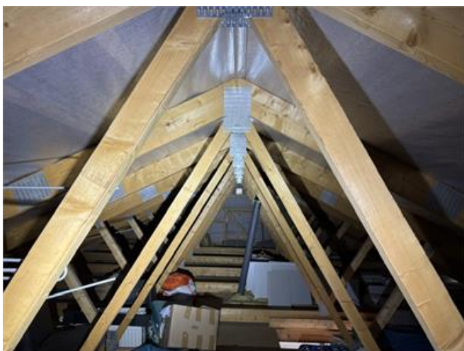
Bilden visar vy av vind (huvudbyggnad).
