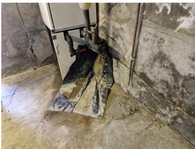
Källare, fuktinträngning och sprucken grundmur.
