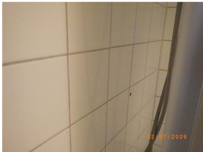
Otättheter i våtzon , (duschrum).
