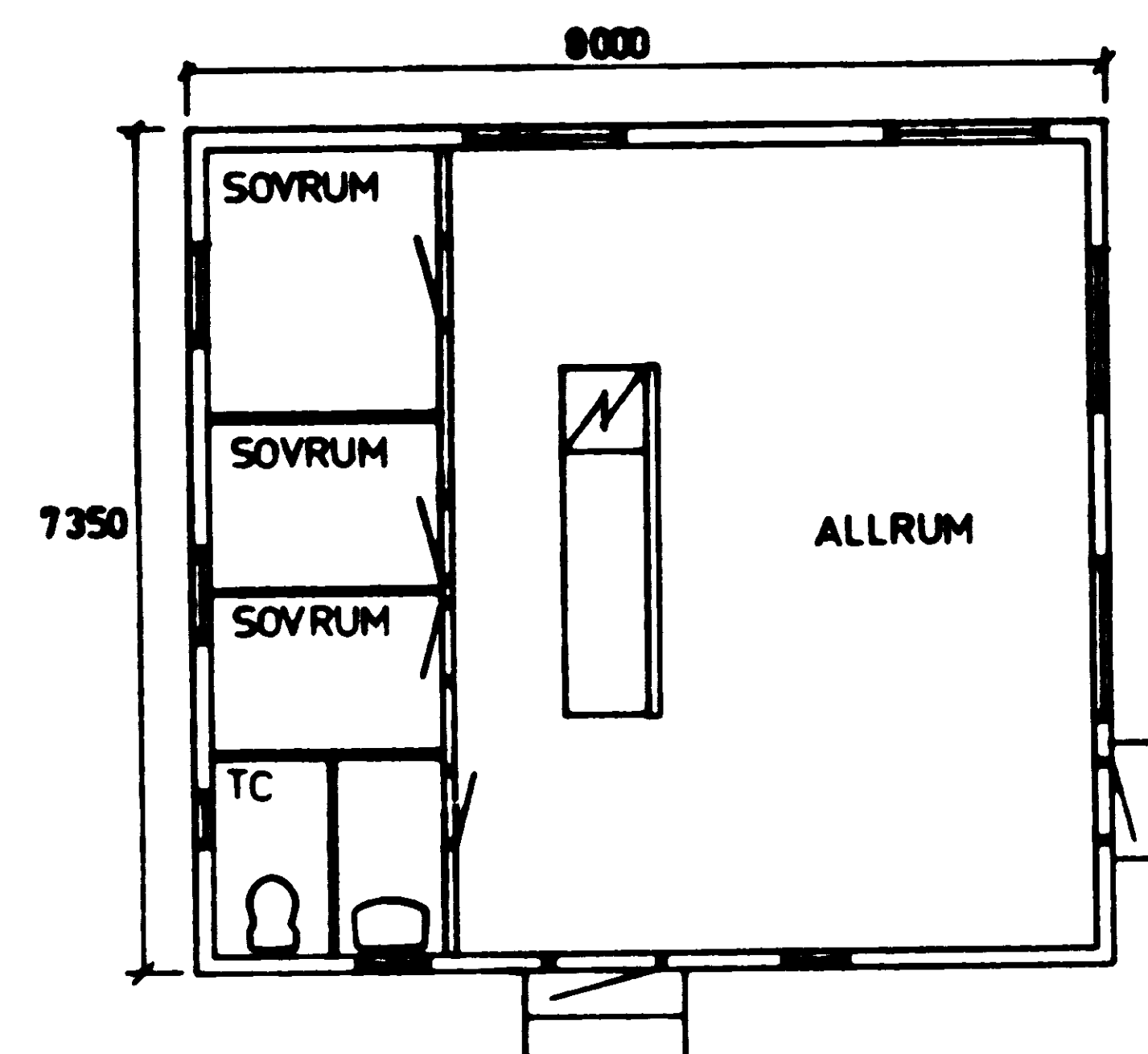
PLAN 1:100
