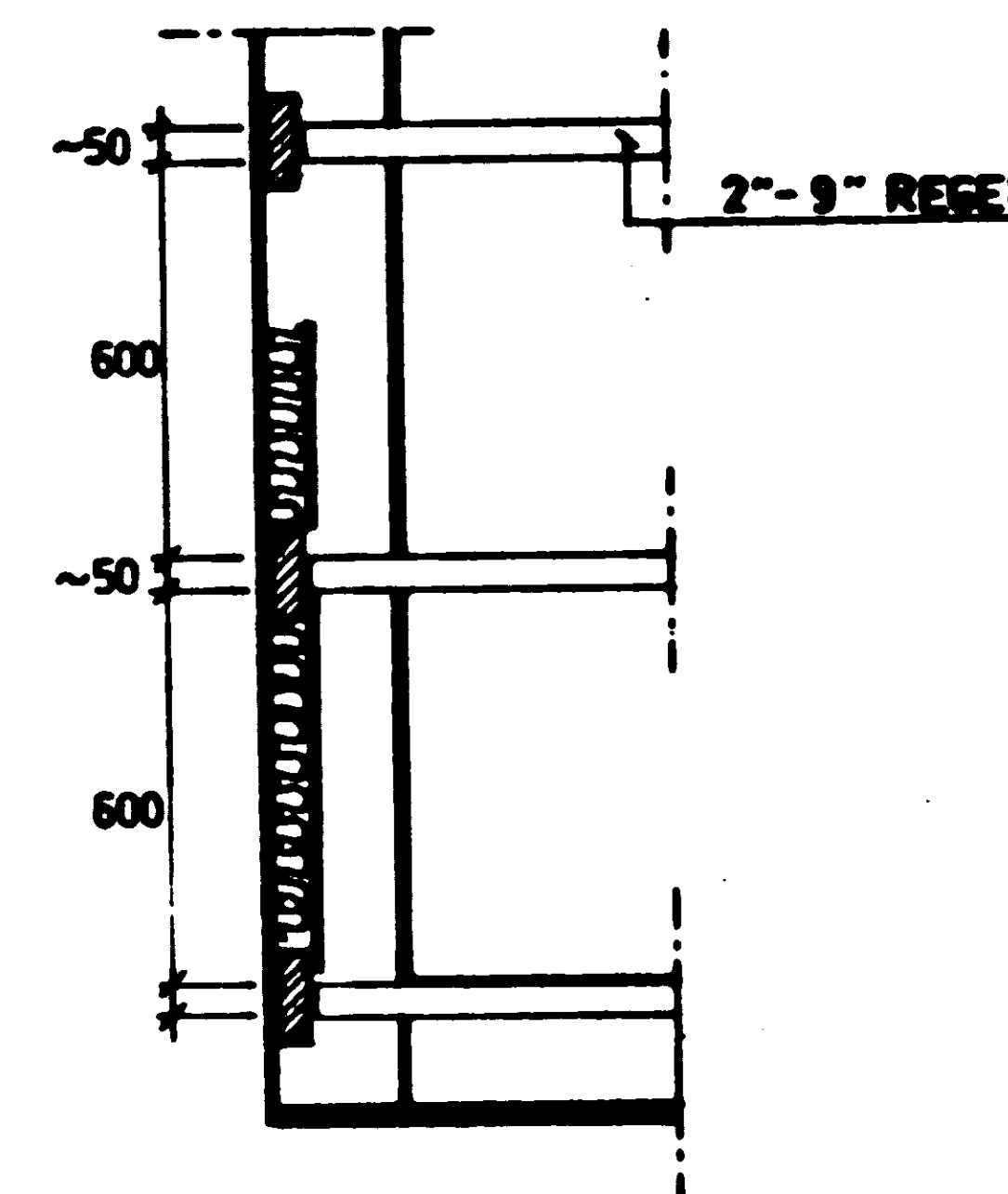
SNITT 1:20
