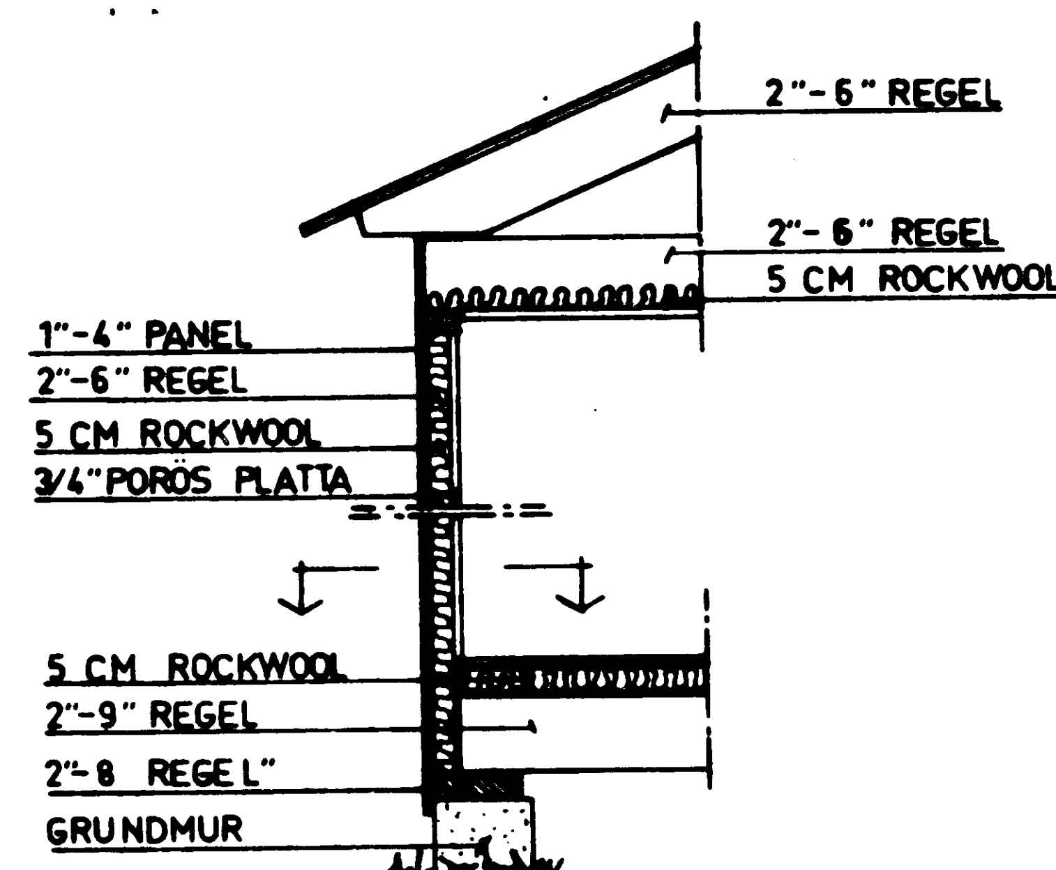
SEKTION 1:20
