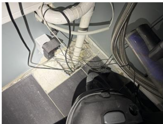
-Under centraldammsugaren har golvet bilats upp för montering av rör. Där av förekommer inget tätskikt på del av golvet. -Mellan tillbyggnad och tvätttrum noterades inget uppvikt fuktskydd mot vägg
