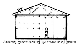
sektion "a-a"
