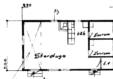
plan 46 m 2 (37+9) tillbyggnad 9 m 2
