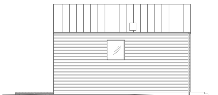
VÄNSTER GAVEL
