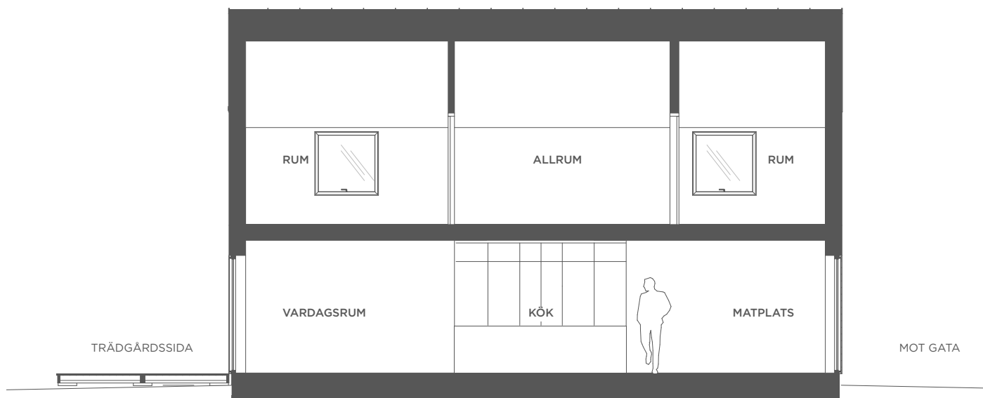
LÄNGDSEKTION
