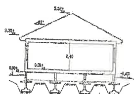
SEKTION PRINCIPITNING
