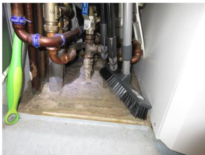
Inget tätskikt/våtrumsmatta på betongklack i tvättstuga.
