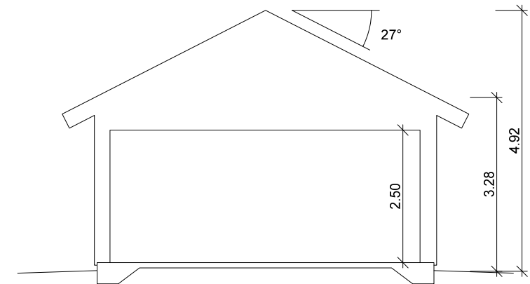
SEKTION A-A
