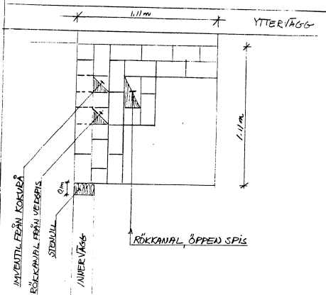
SEKCTION: SKALA 1:100
