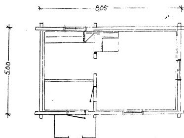
PLAN SKALA 1:100
