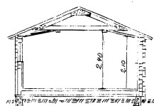
SEKCTION: SKALA 1:100
