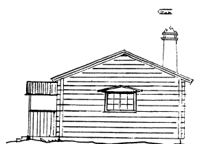
FASAD ÖSTER
