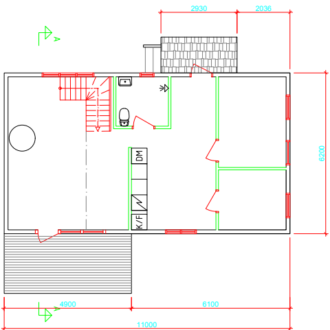
PLAN 1 (BEFINTLIG)
