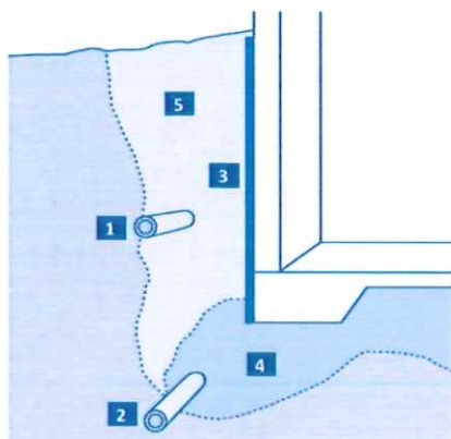
Fuktspärre med asfaltstrykning
