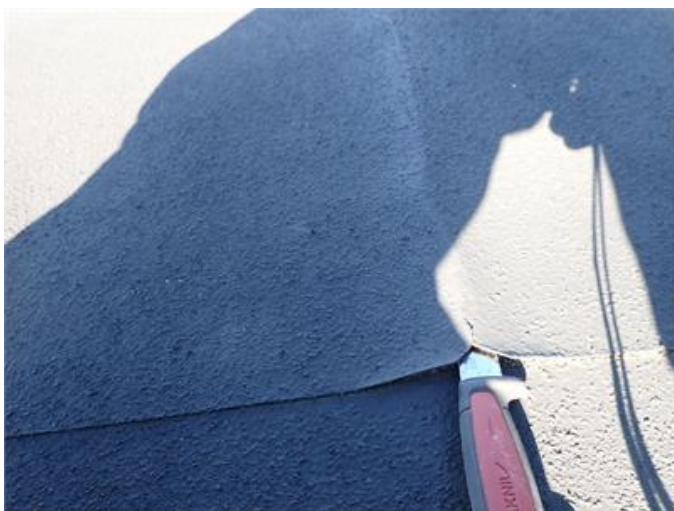
Exempel på otätet i takpappens skarv.
