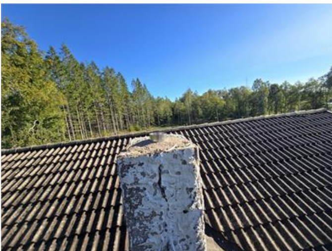
Tak: Skorsten har färgsläpp samt sprickor, väderskydd finns ej.
