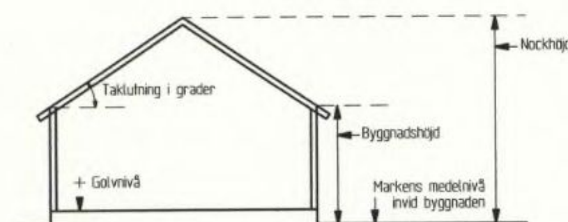
Principskiss över hur höjder och taktvinkel beräknas.
