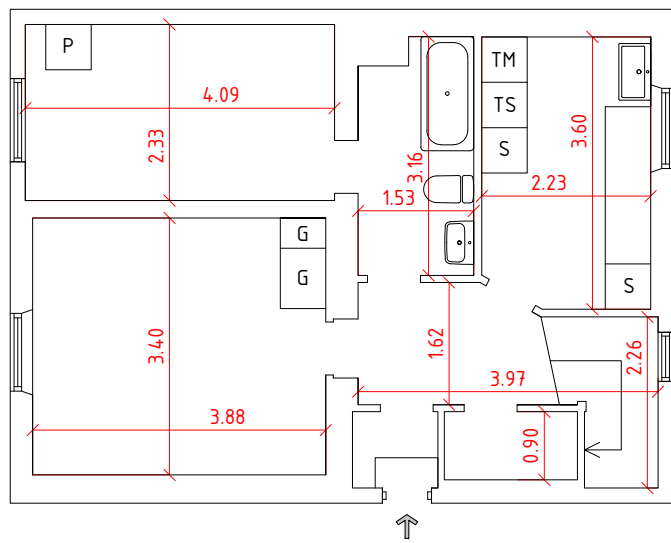
KÄLLARPLAN
