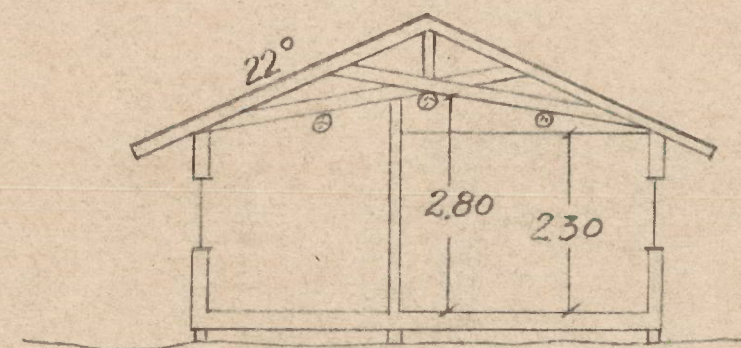
Sektion
