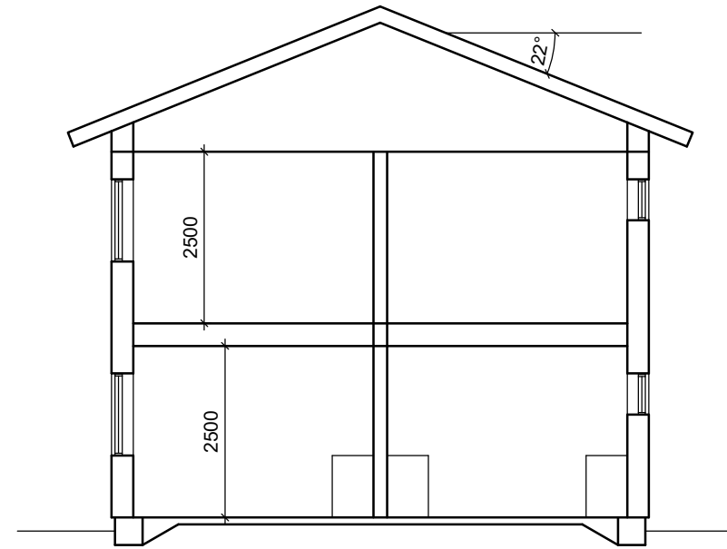
PRINCIPSEKTION A-A
