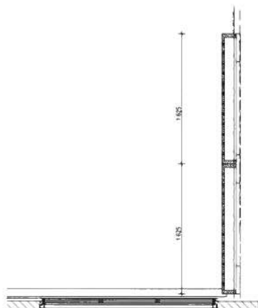
Tvärsektion
