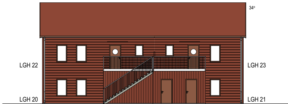
FASAD ENTRÉ
