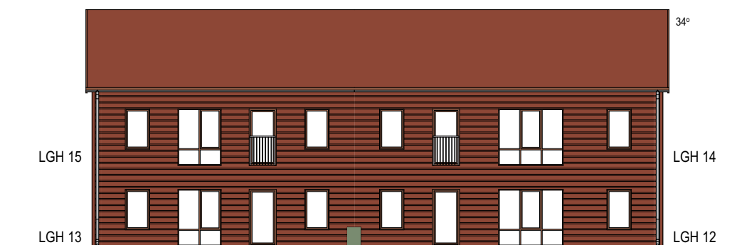
FASAD TRÄDGÅRD
