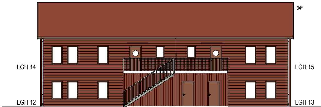
FASAD ENTRÉ
