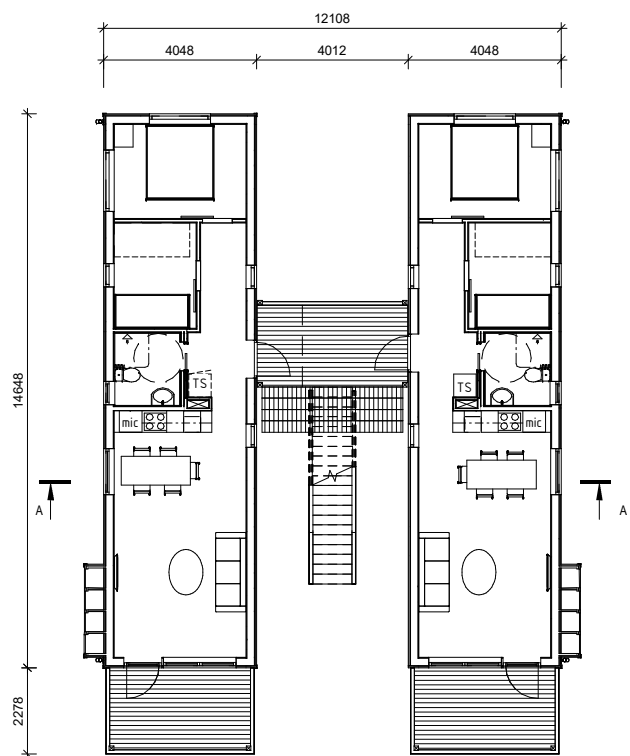
Plan 1 Bygglov 1: 100
