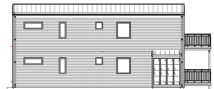
Fasad mot Väster 1 1: 100
