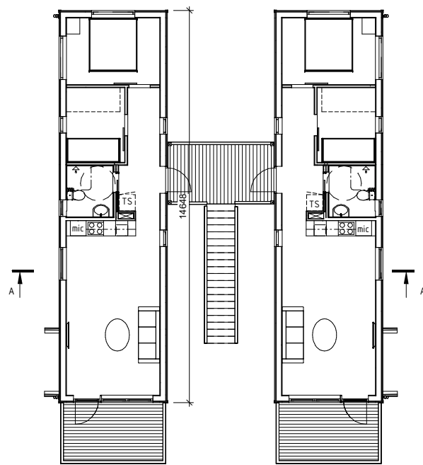
Plan 2 Bygglov 1: 100
