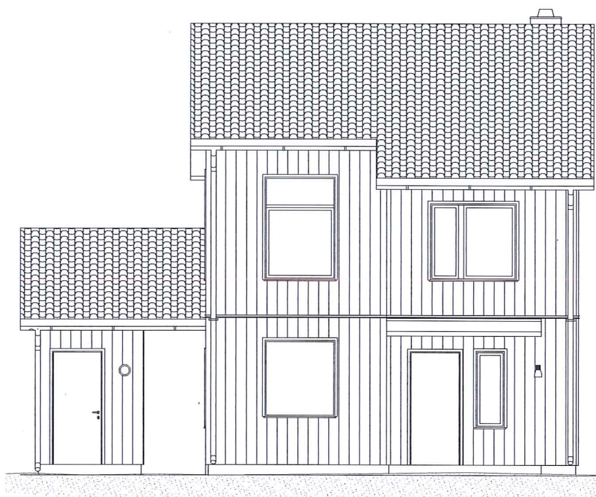
FASAD MOT GATA
