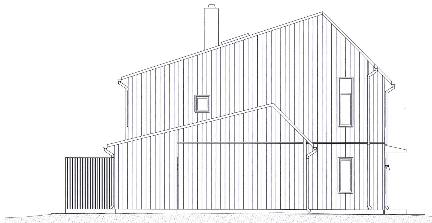
FASAD MOT CARPORT
