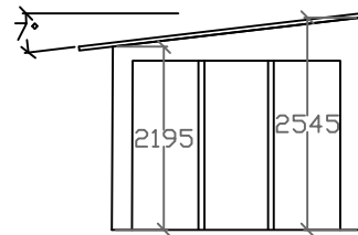
SEKTION TILLBYGGNAD
