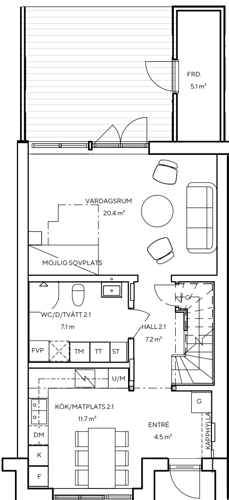
Entréplan – 53,6 kvm
