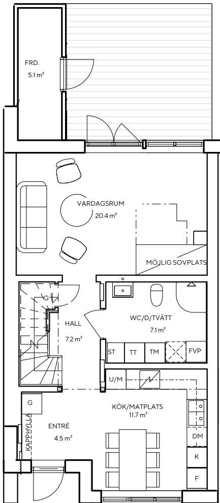
Entréplan - 53,6 kvm
