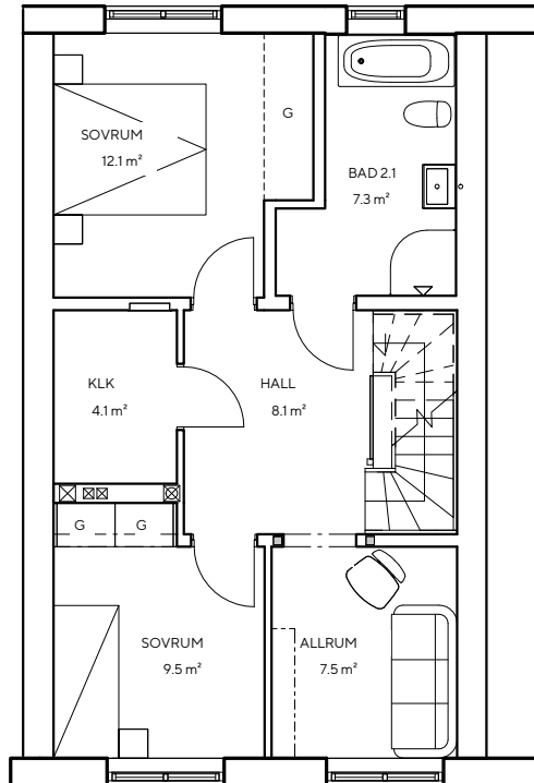
Plan 2 – 55,3 kvm
