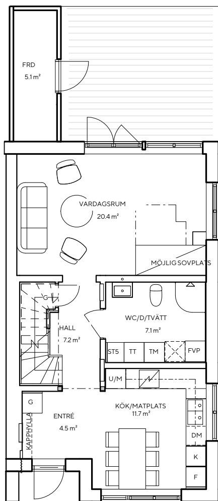
Entréplan – 53,6 kvm
