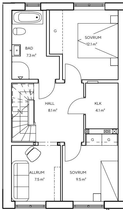
Plan 2 – 55,3 kvm
