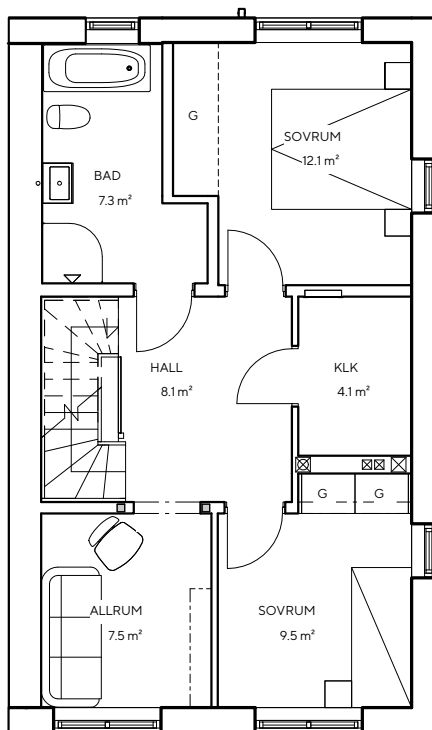
Plan 2 – 55,3 kvm
