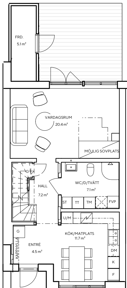
Entréplan – 53,6 kvm
