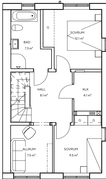
Plan 2 – 55,3 kvm
