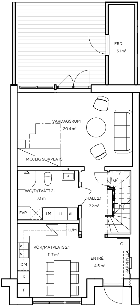
Entréplan – 53,6 kvm
