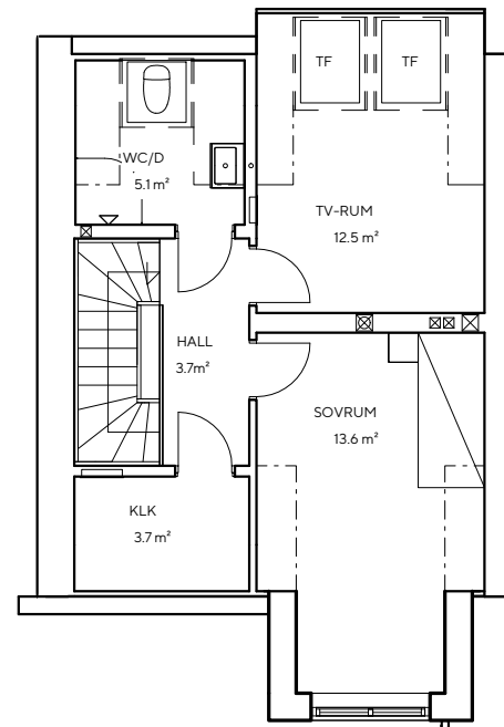
Plan 3 - 41,7 kvm
