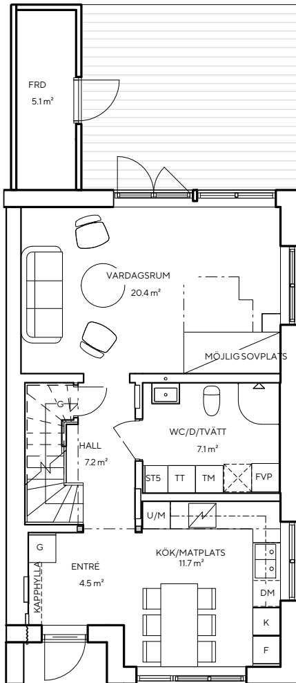
Entréplan – 53,6 kvm
