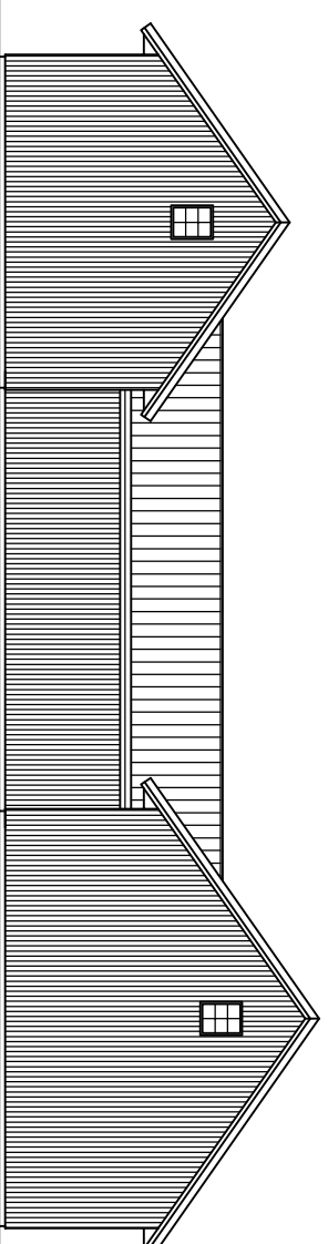
FASAD MOT NORDÖST
