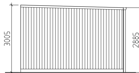
FASAD 3
