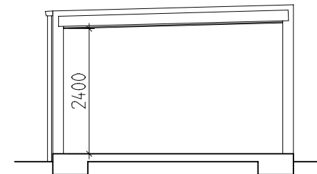
SEKTION
