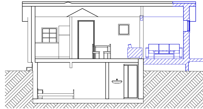
Sektion B-B 1:100
