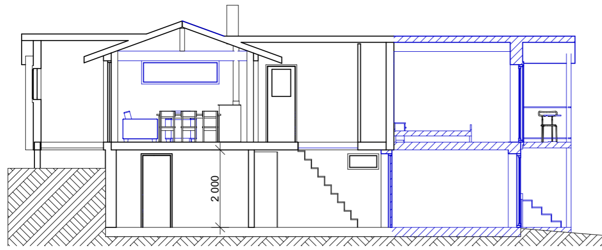
Sektion A-A 1:100
