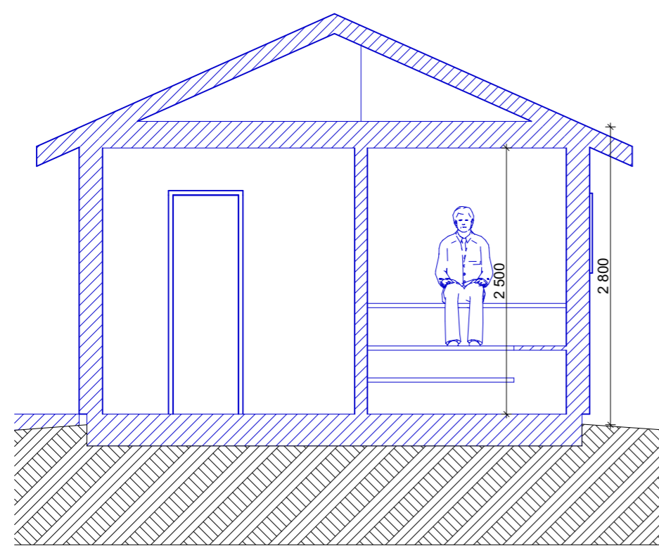
Sektion A'-A' 1:50
