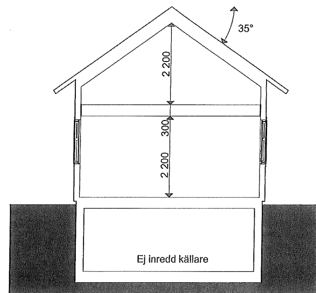
Sektion A-A
