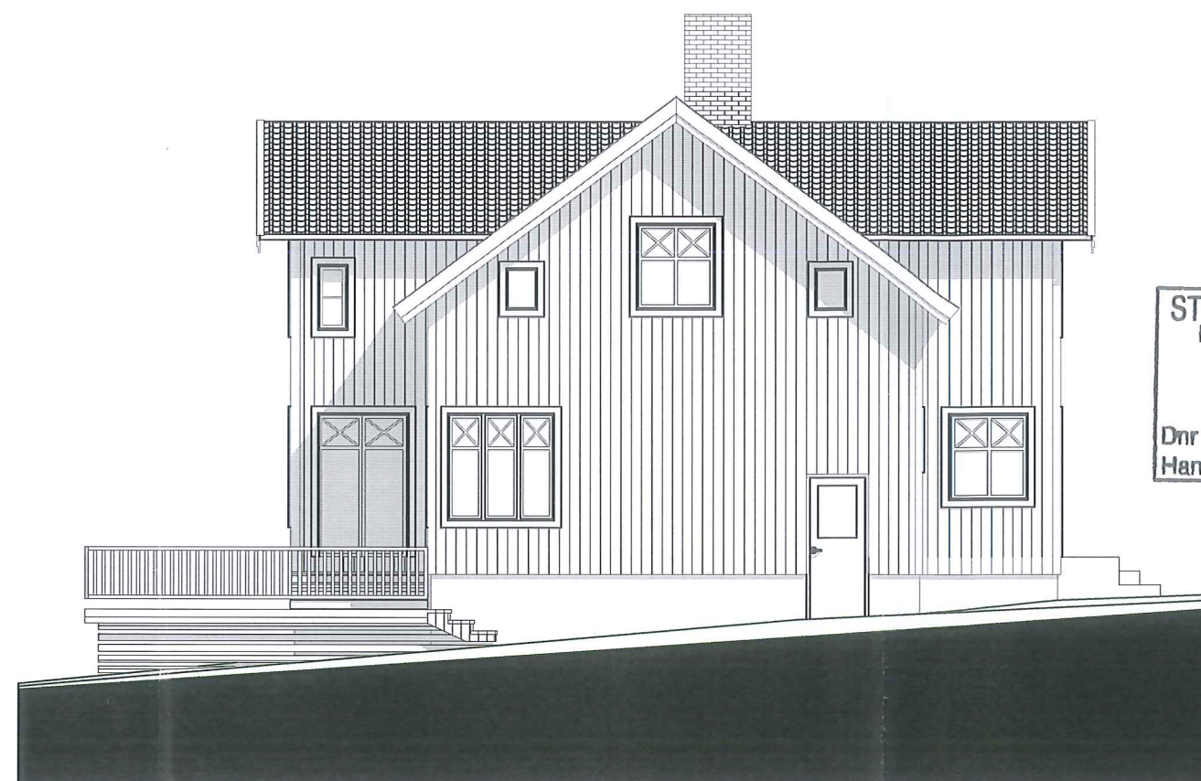
Fasad Söder
