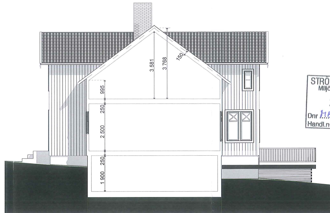
Sektion A-A
