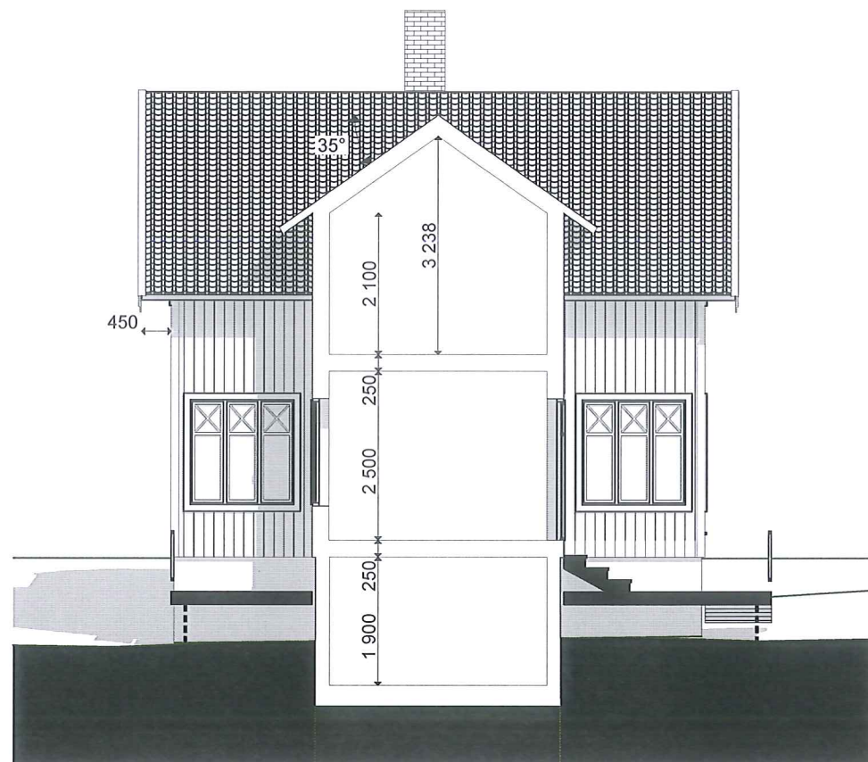
Sektion B-B
