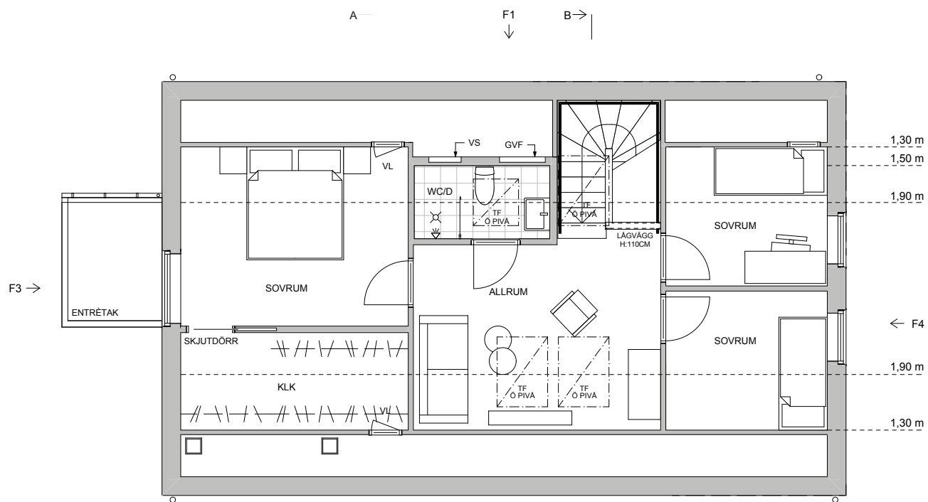
PLAN 2 (skala 1:100)
