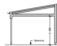
Sektion C (skala 1:200)
