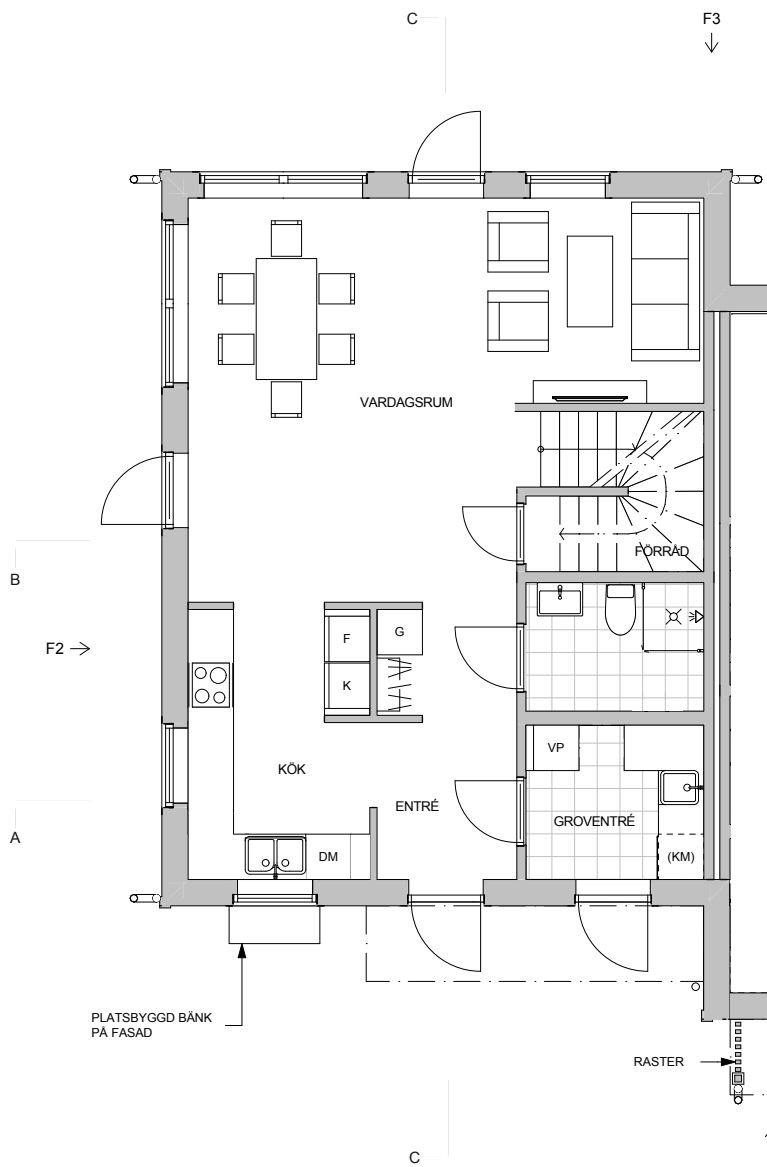
PLAN 1 (skala 1:100)
