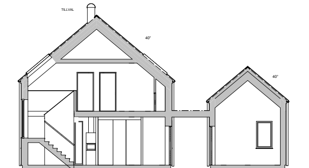
Sektion (skala 1:200)
