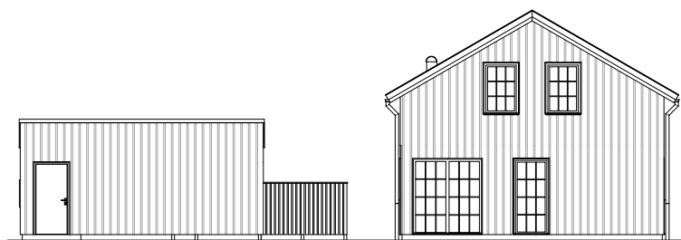
Fasad 4 (skala 1:200)
