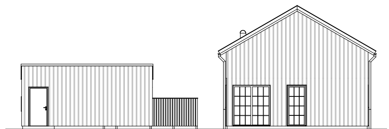
Fasad 4 (skala 1:200)
