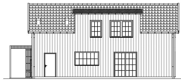
Fasad 2 (skala 1:200)
