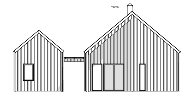
Gavelfasad (skala 1:200)
