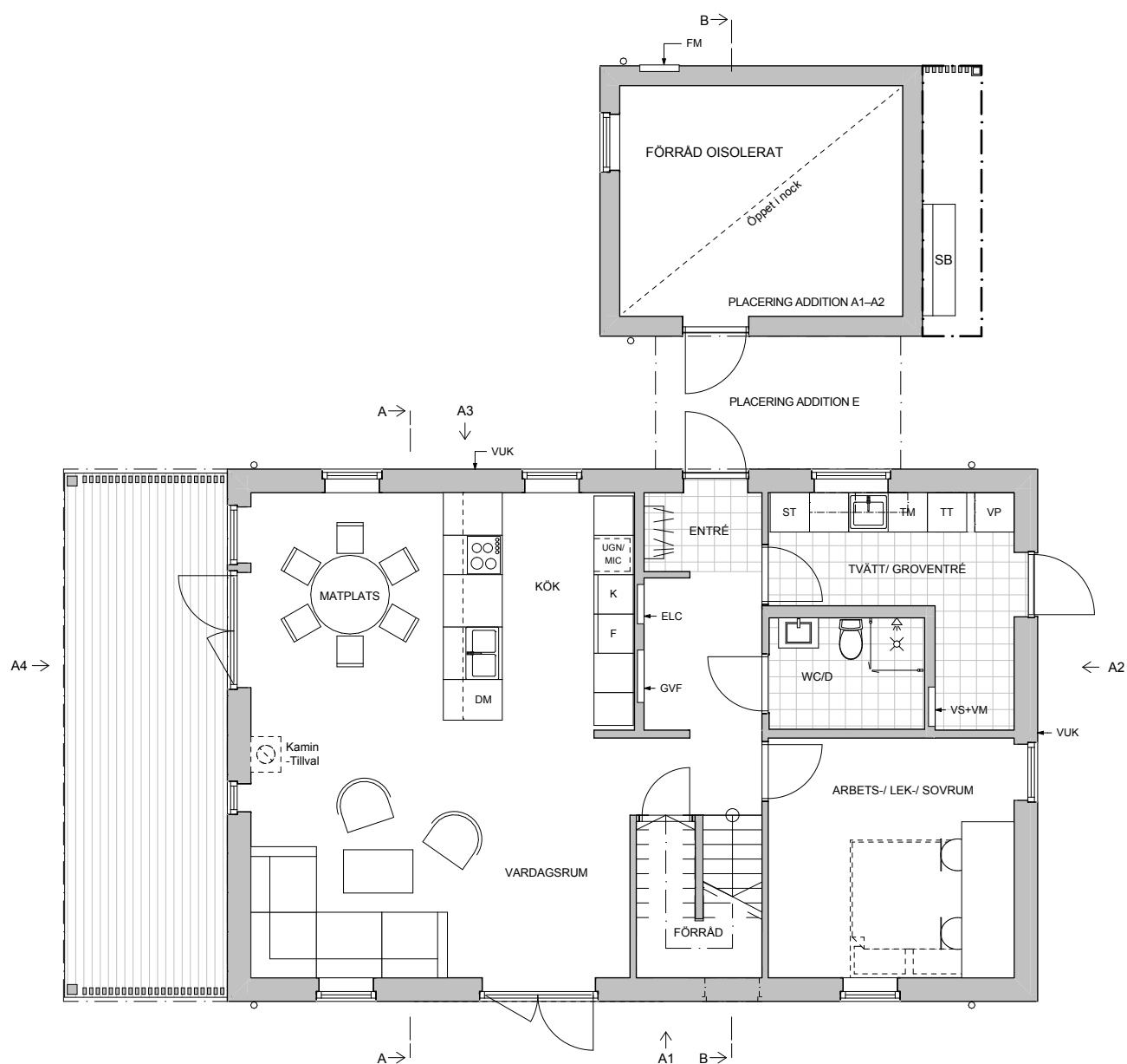
PLAN 1 (skala 1:100)
