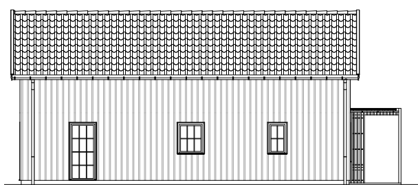
Fasad 1 (skala 1:200)
