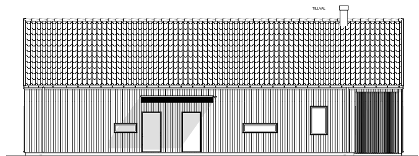
Entréfasad (skala 1:200)
