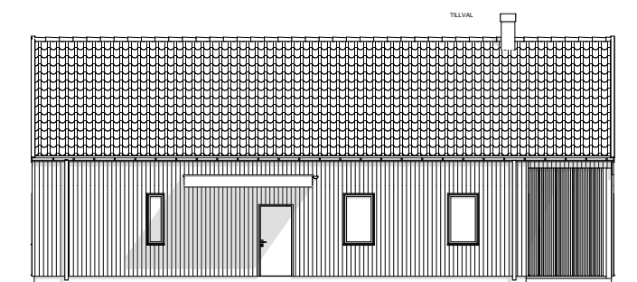
Entréfasad (skala 1:200)
