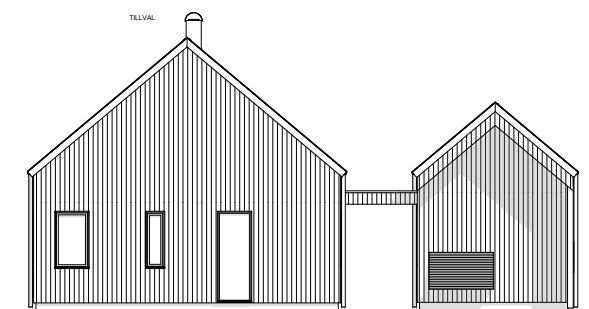
Gavelfasad (skala 1:200)
