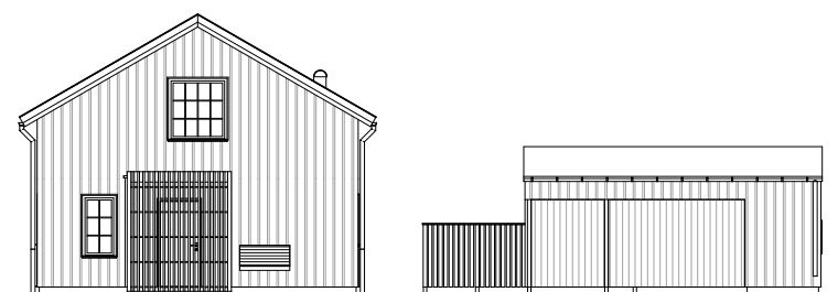
Fasad 3 (skala 1:200)
