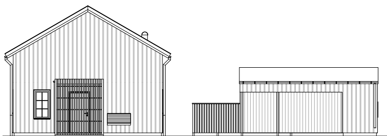
Fasad 3 (skala 1:200)
