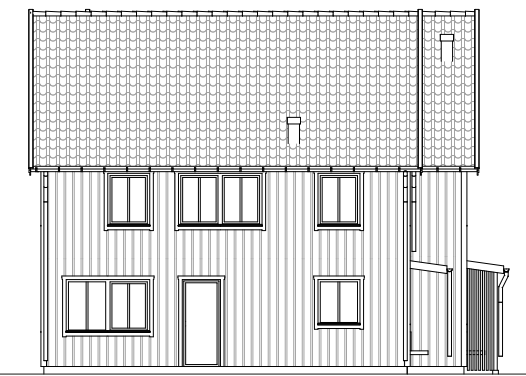
Fasad 2 (skala 1:200)
