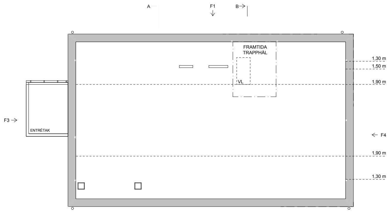
PLAN 2 (skala 1:100)
