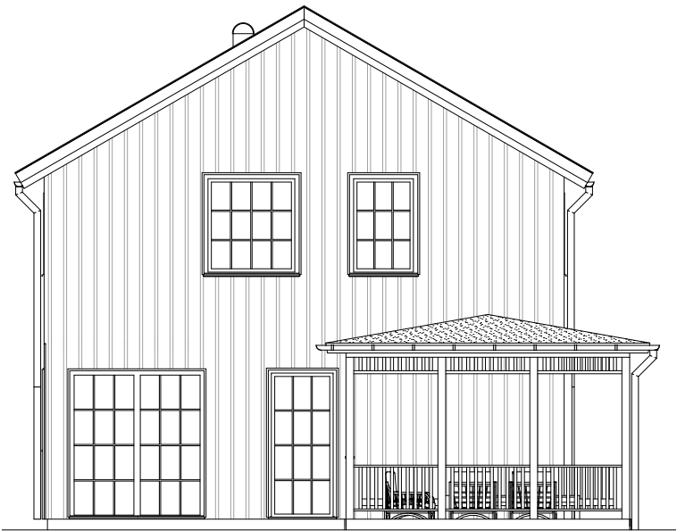
Fasad 4 (skala 1:100)
