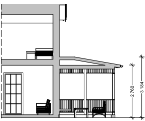
Sektion D (skala 1:200)
