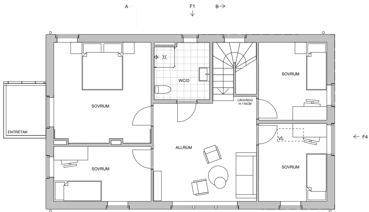
PLAN 2 (skala 1:100)
