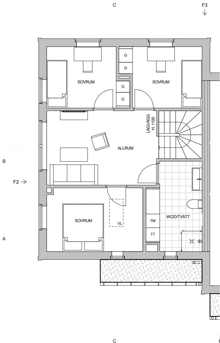
PLAN 2 (skala 1:100)
