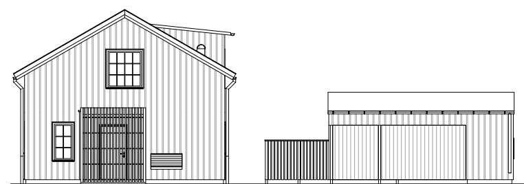
Fasad 3 (skala 1:200)
