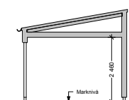
Sektion C (skala 1:200)
