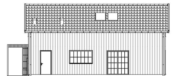
Fasad 2 (skala 1:200)
