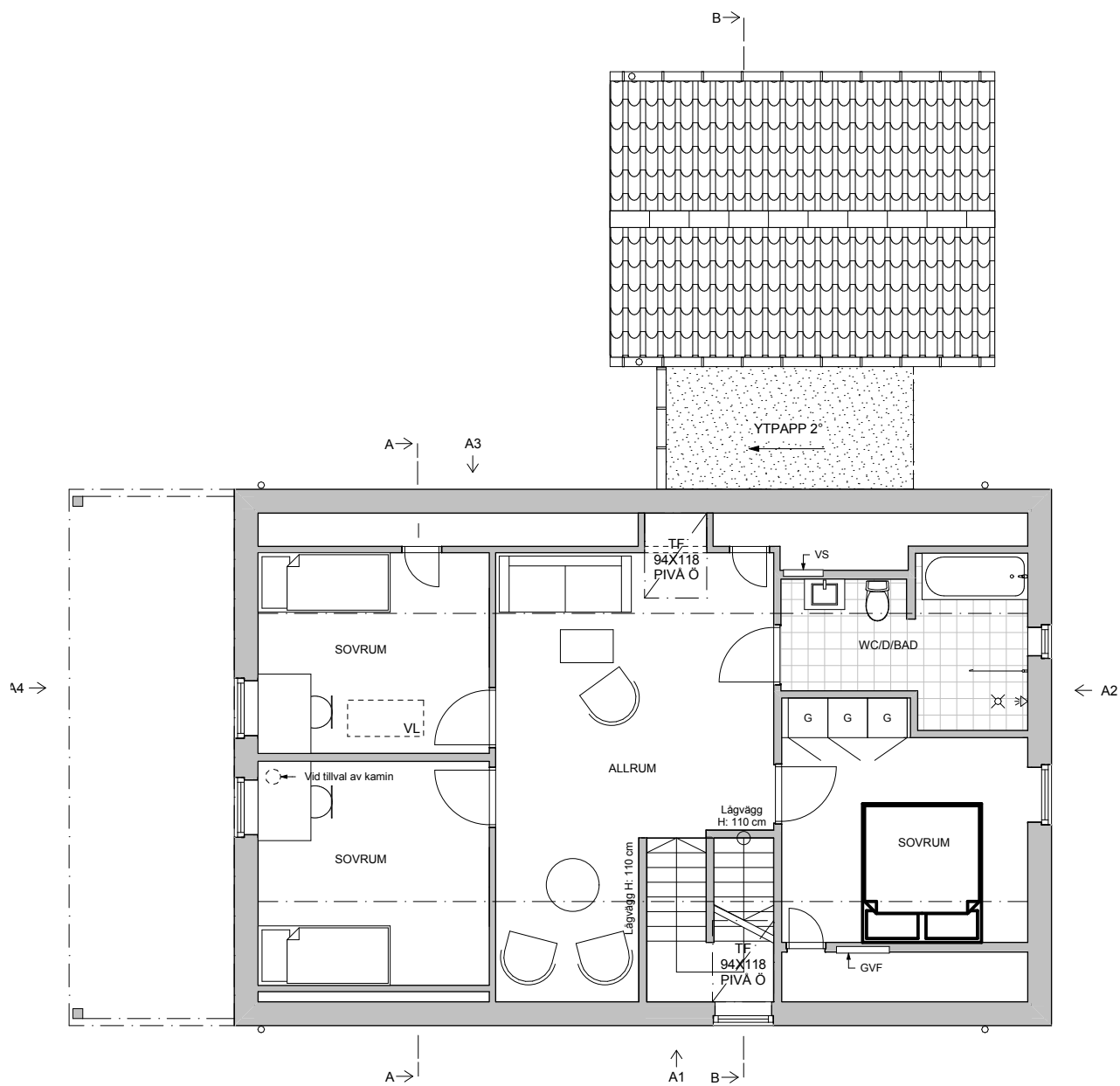
PLAN 2 (skala 1:100)
