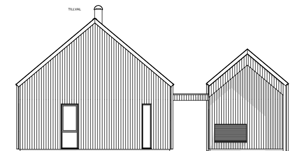
Gavelfasad (skala 1:200)
