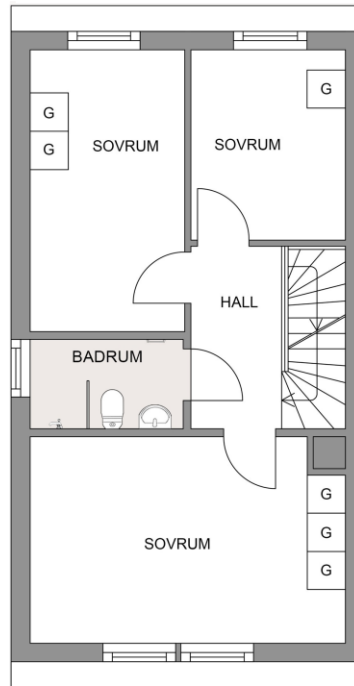
VINDSPLAN
