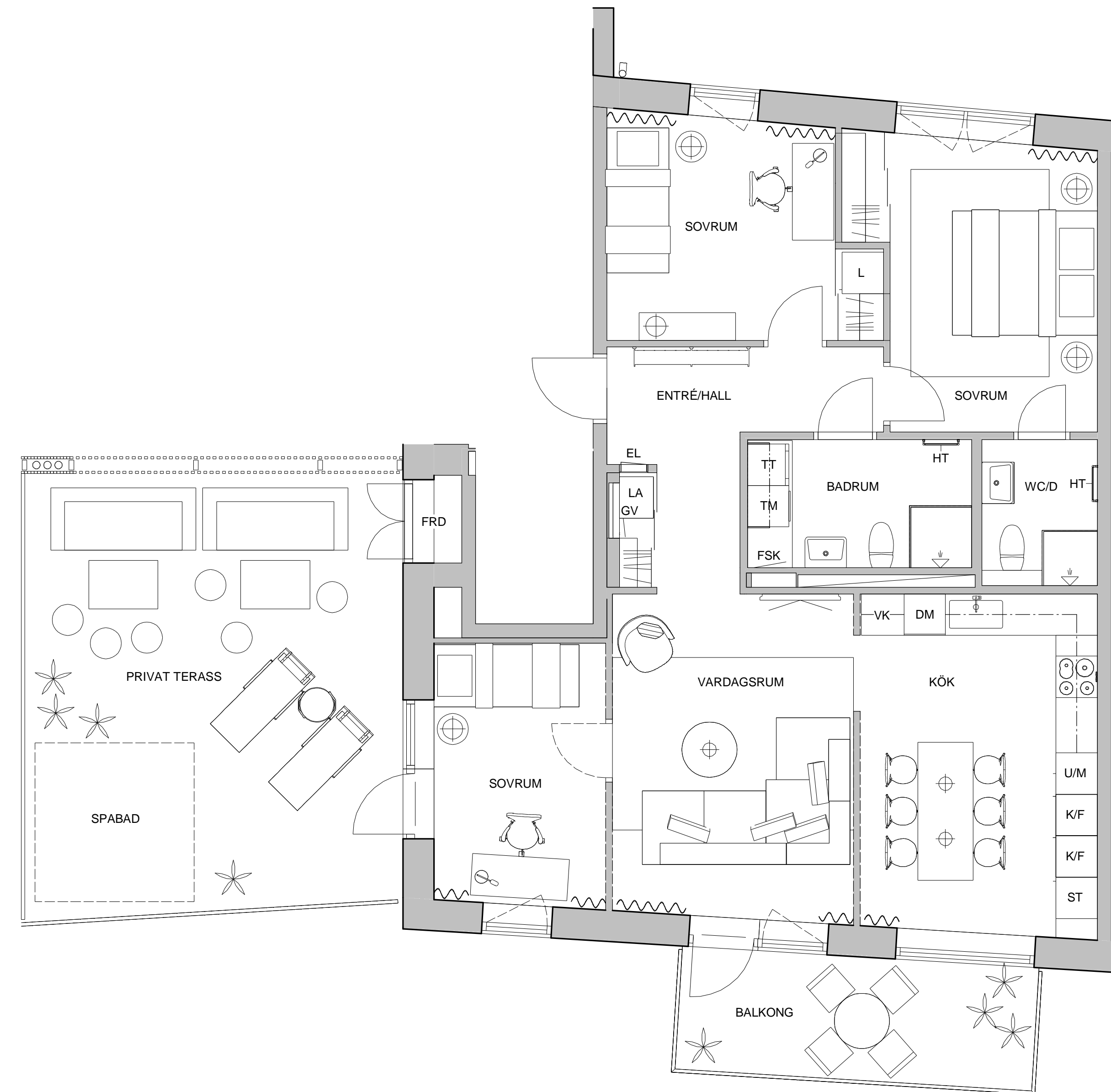
MÖBLERINGSPLAN LGH A-1501 - ALT.4
