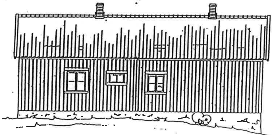
Soldattorpet Dala. Ritning från 1911.
