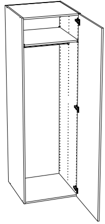
GARDEROB Ett hyllplan och en klädstång.
