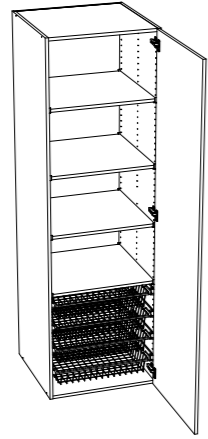
LINNESKÅP Fyra hyllplan och fyra trådbackar.
