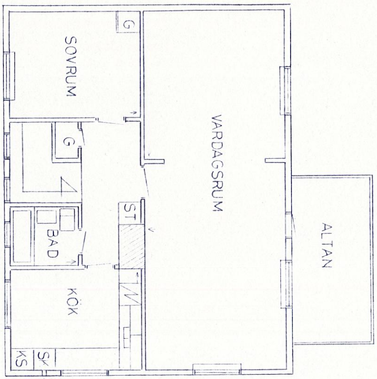
VÅNINGSPLAN
