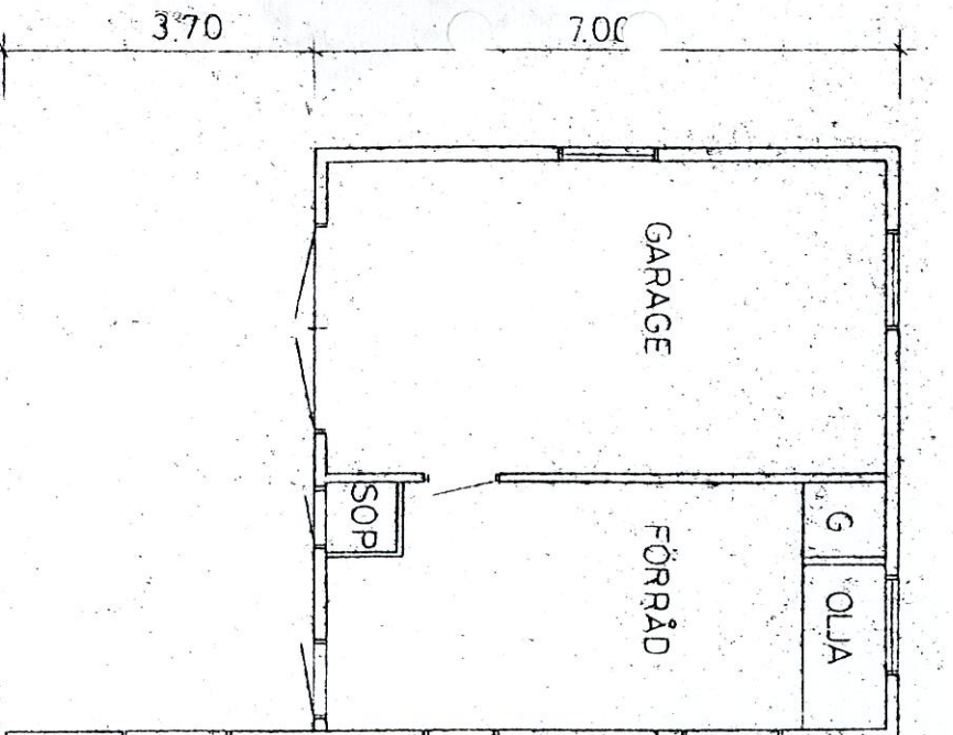
ENTREVÅNING 7.00 TILLBYGGNAD
