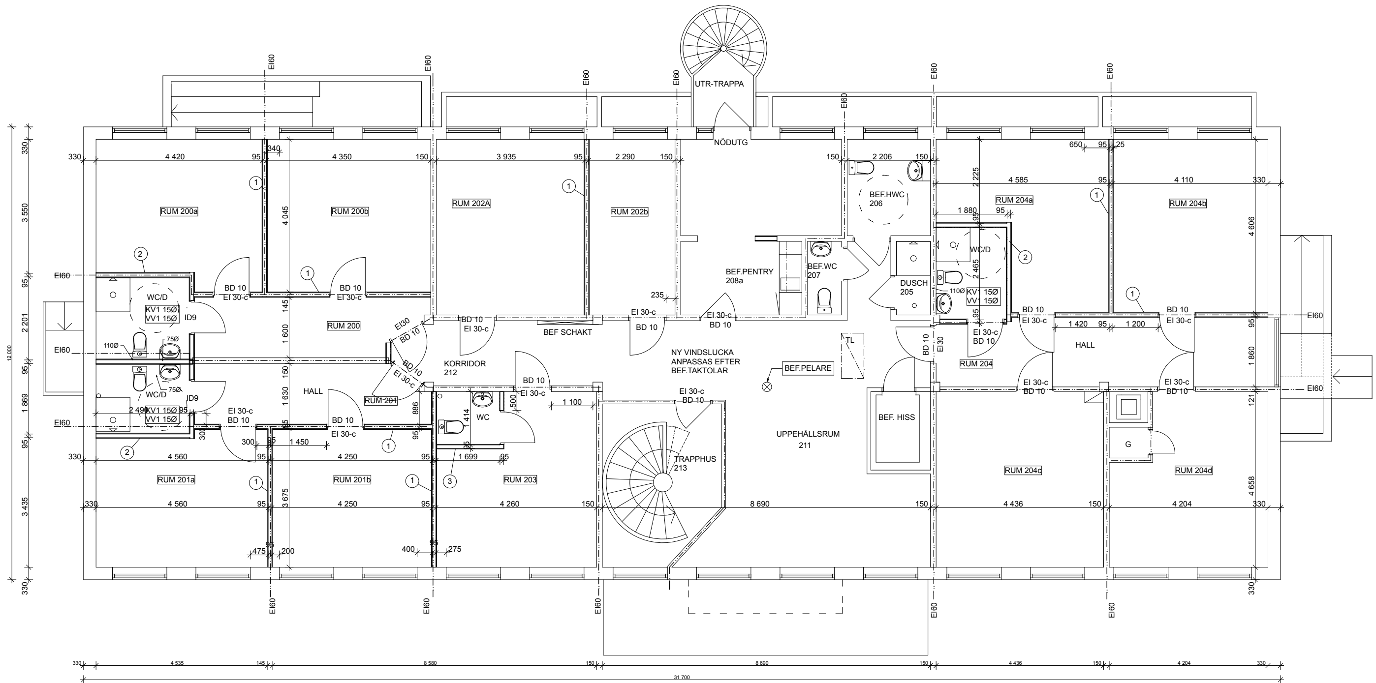
PLAN OVANVÅNING SKALA 1:100 A3, 1:50 A1
