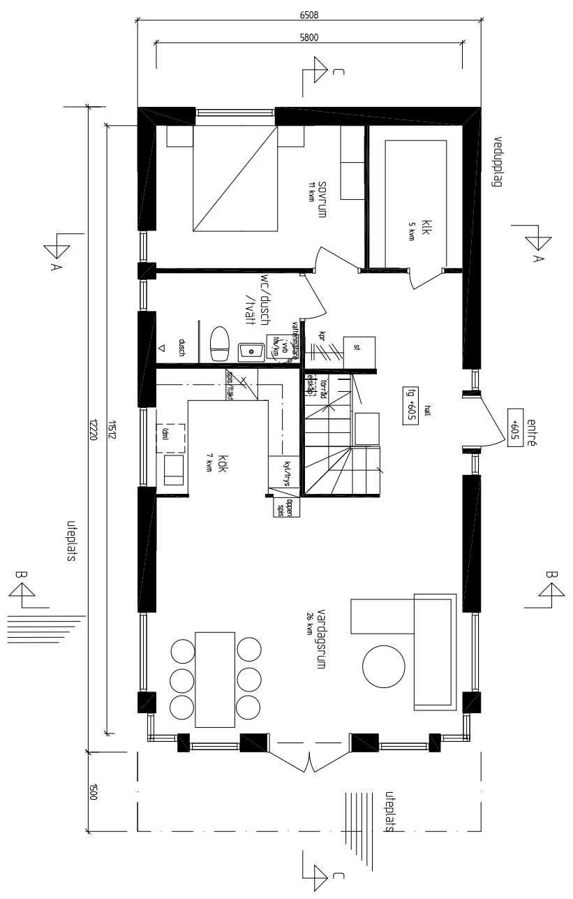
BOTTEPLAN LGH YTA 66,7 kvm
