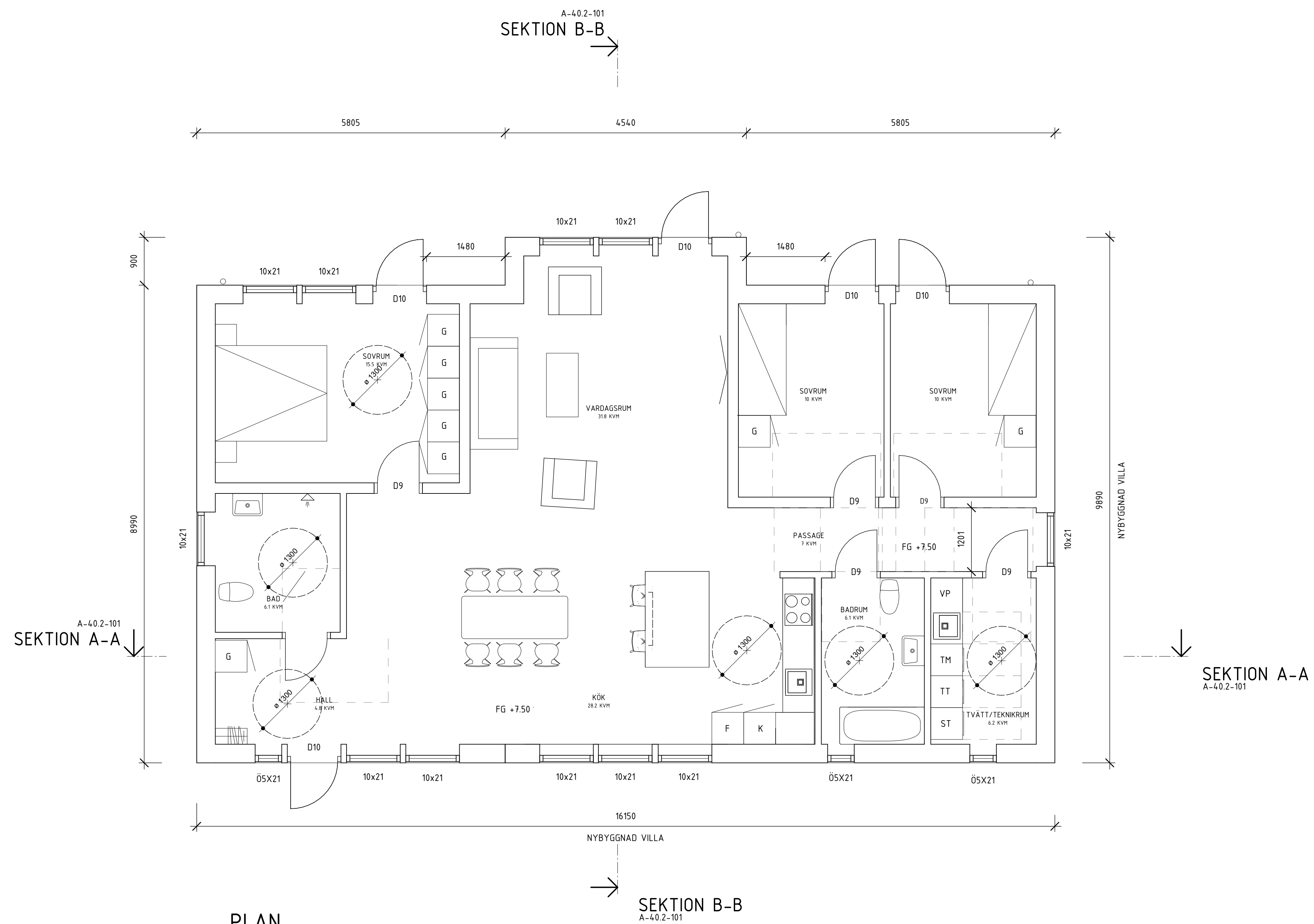
PLAN 1 : 50
