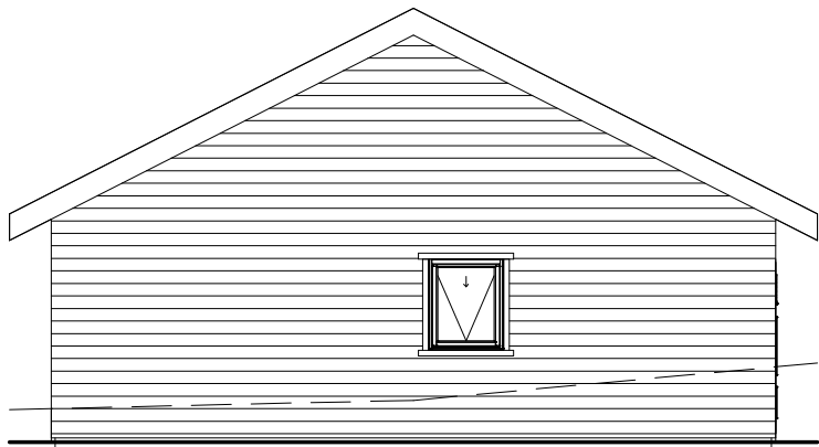
2 Söder 1 : 100
