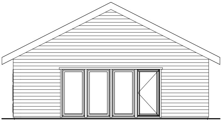
4 Väster 1 : 100
