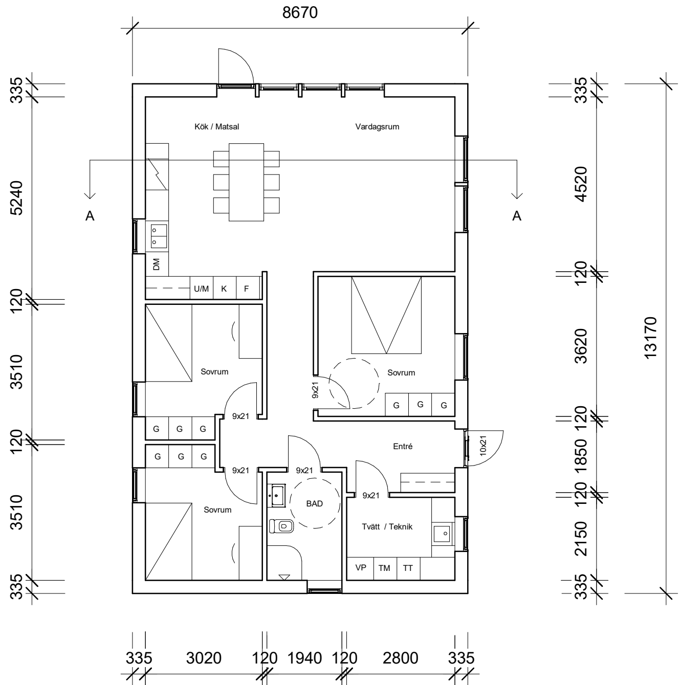
1 Planlösning 1 : 100
