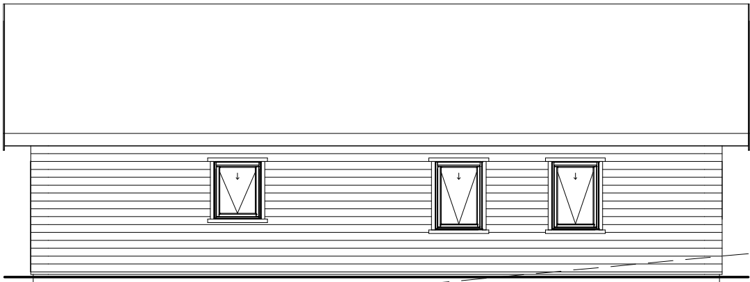
4 Väster 1 : 100
