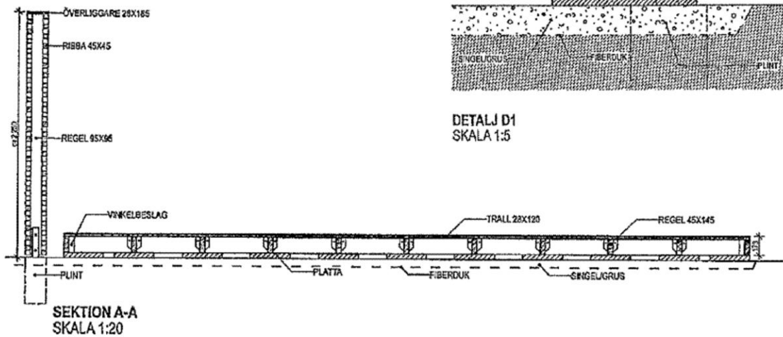
Figur 4 RITNING MARKTERASS 3(3)
