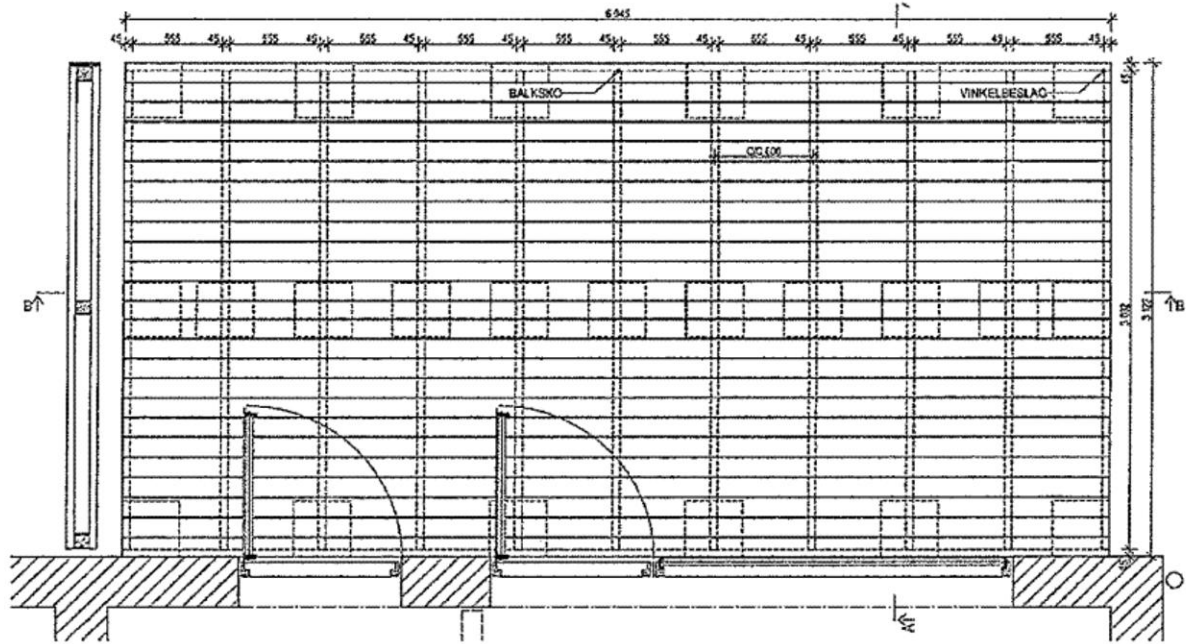
PLAN SKALA 1:20
