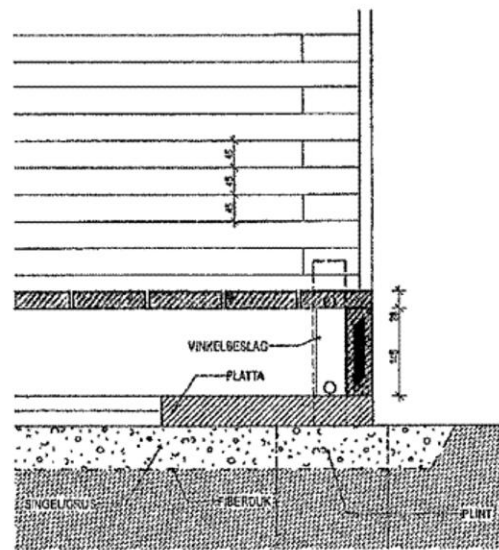
DETALJ D1 SKALA 1:5
