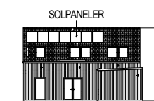
FASAD MOT SYDOST
